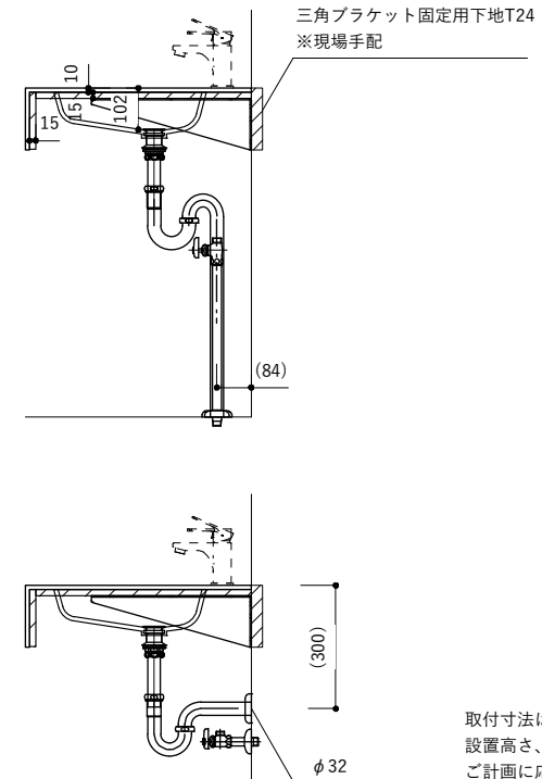
【断面図】
