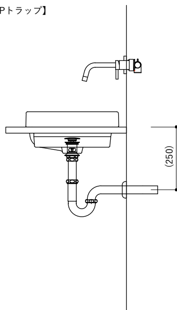
【側面図・Pトラップ】
