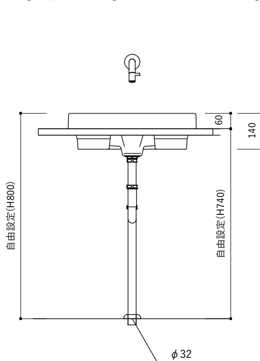
【正面図・Sトラップ】
