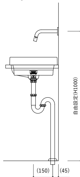
【側面図・Sトラップ】
