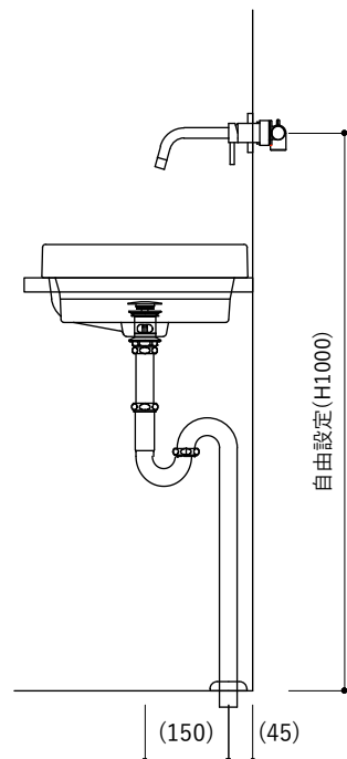
【側面図・Sトラップ o 】
