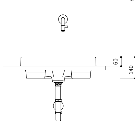
【正面図・Pトラップ】
