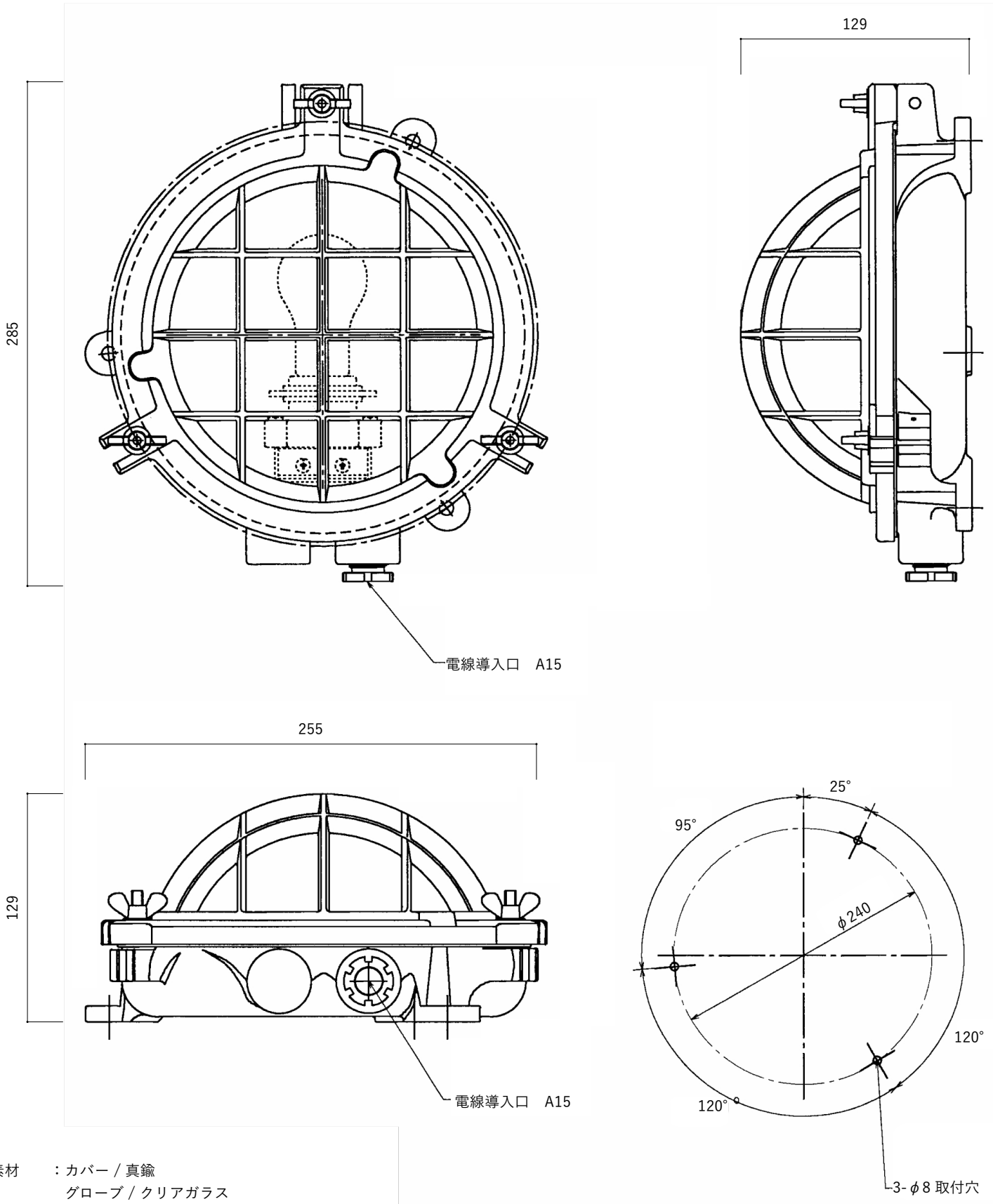
【取付面 寸法図】
