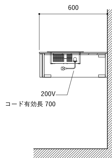
コンロ断面
