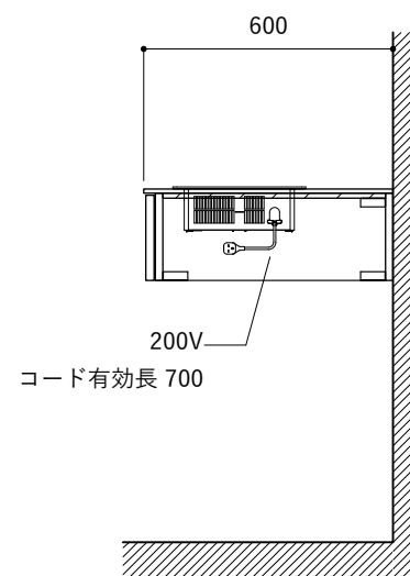
コンロ断面
