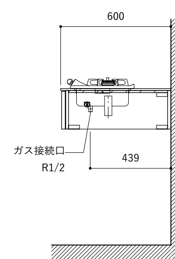
コンロ断面
