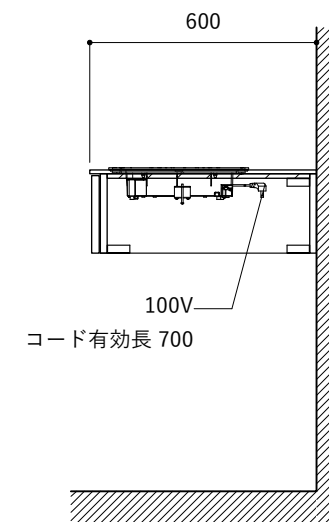
コンロ断面
