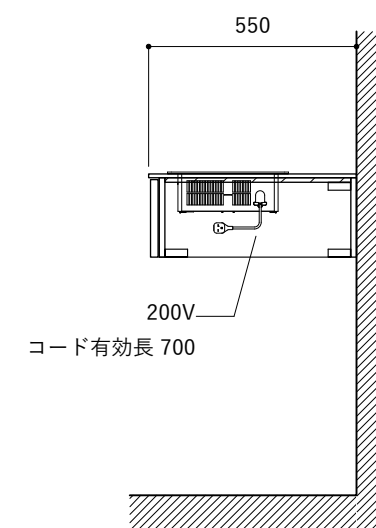
コンロ断面
