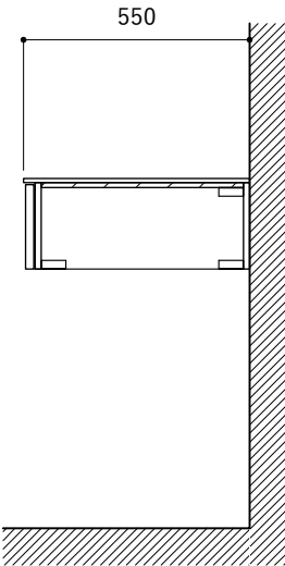
コンロ断面
