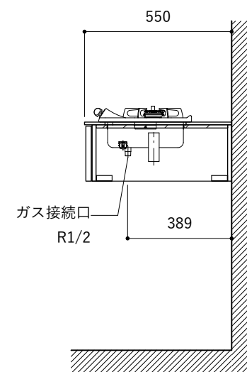
コンロ断面
