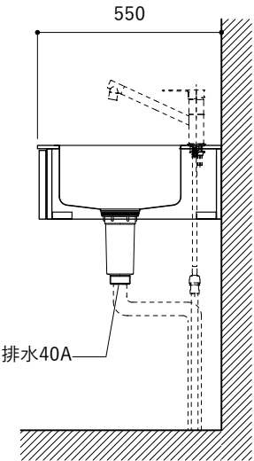
シンク断面
