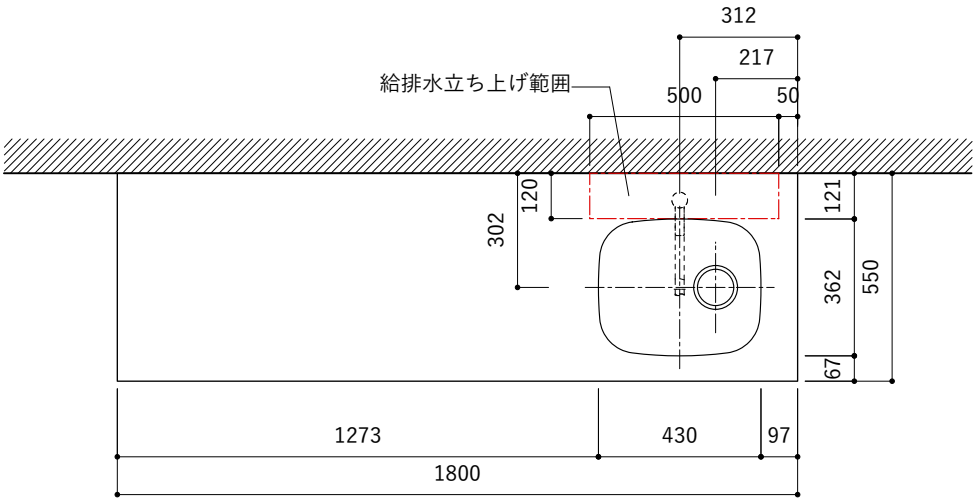
平面
