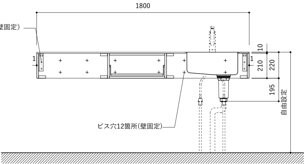
断面
