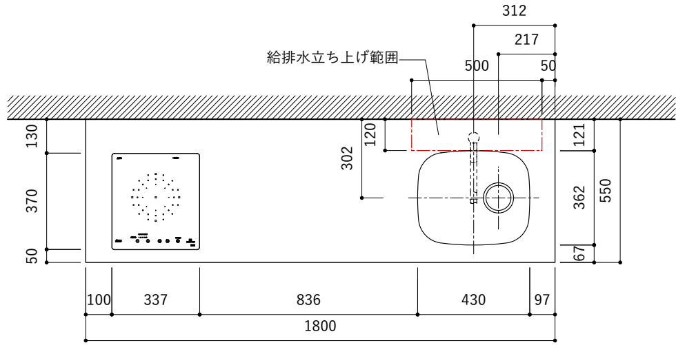
平面
