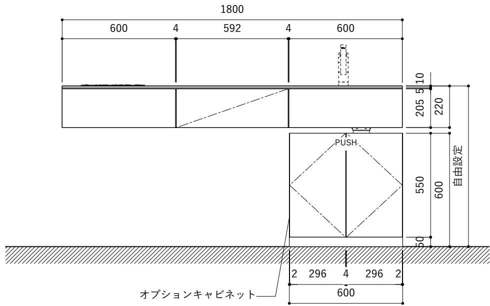
正面
