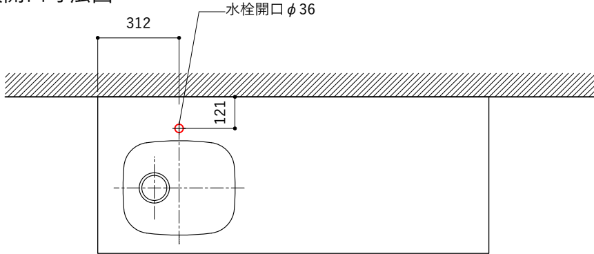
天板開口寸法図
