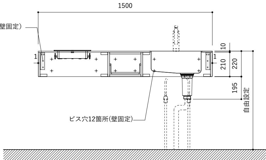
断面
