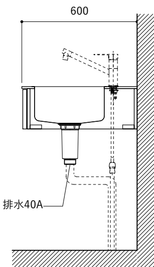
シンク断面
