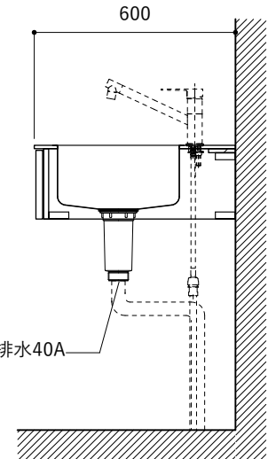
シンク断面
