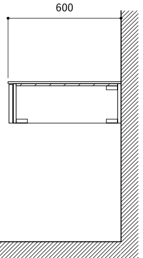
コンロ断面
