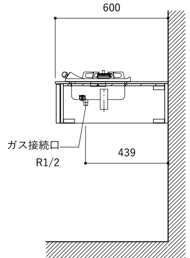
コンロ断面
