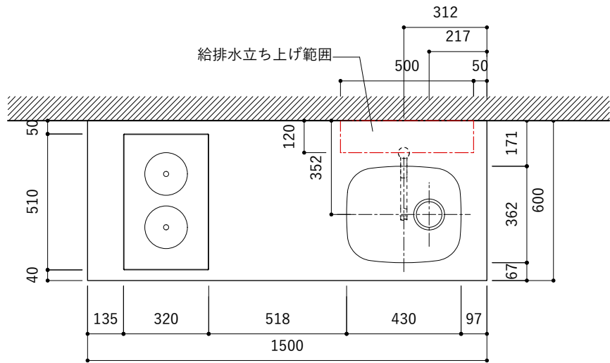
平面
