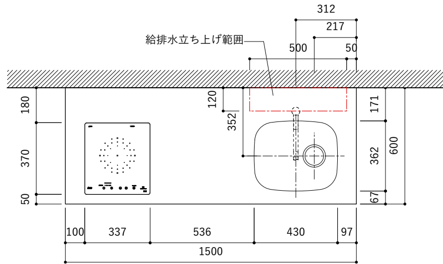
平面
