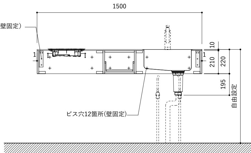
断面
