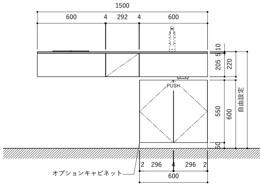
正面
