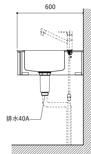
シンク断面
