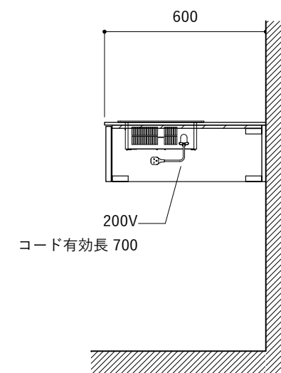
コンロ断面
