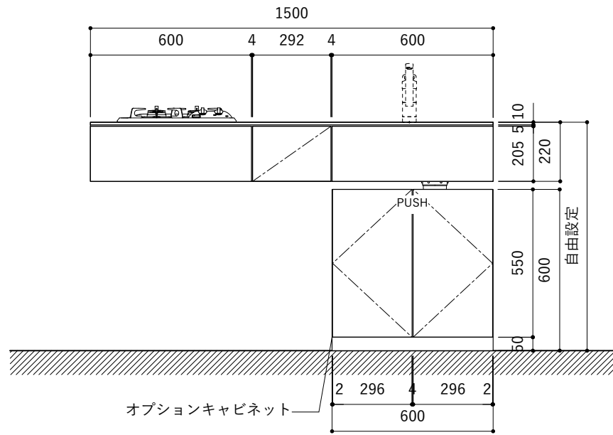
正面
