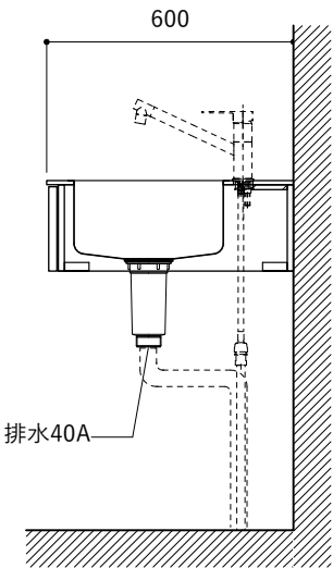
シンク断面
