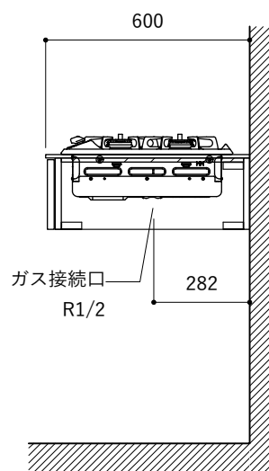
コンロ断面
