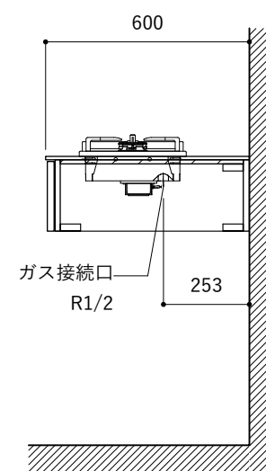
コンロ断面
