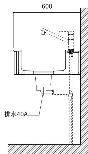
シンク断面
