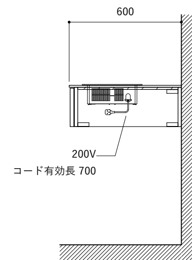
コンロ断面
