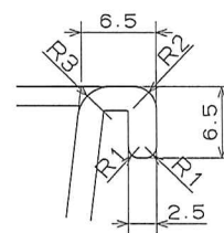
E部詳細 (S=2/1)
