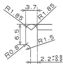
D部詳細 (S=2/1)
