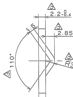
B部詳細 (S=2/1)
