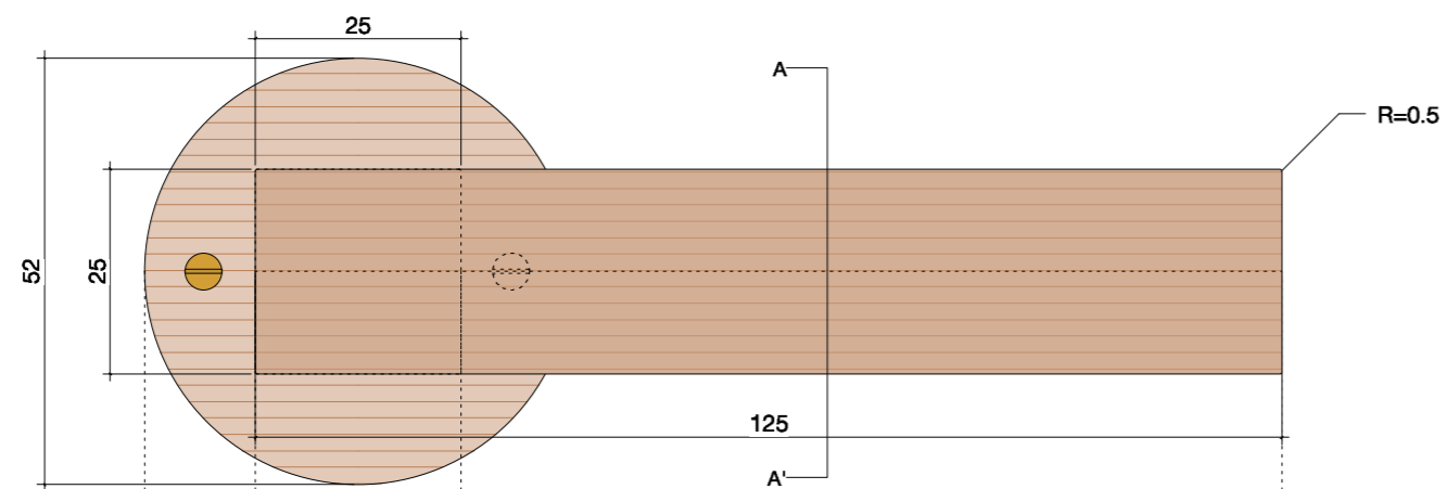
正面図
