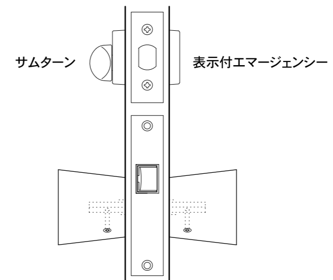
間仕切錠
