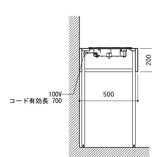
コンロ断面
