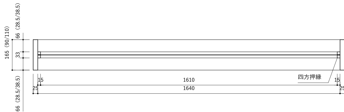
横断面図
