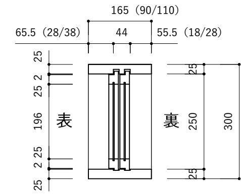
縦断面図
