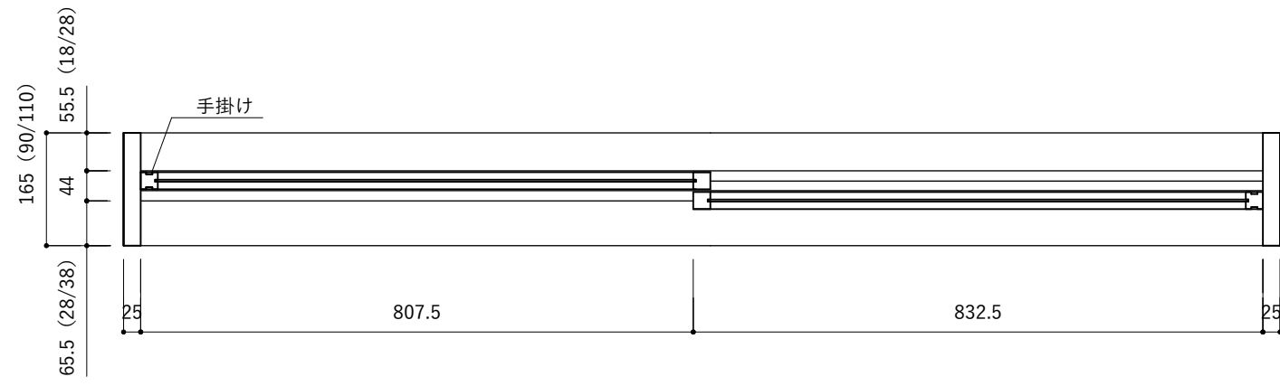
横断面図
