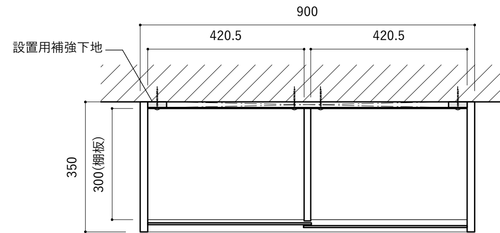
平断面図
