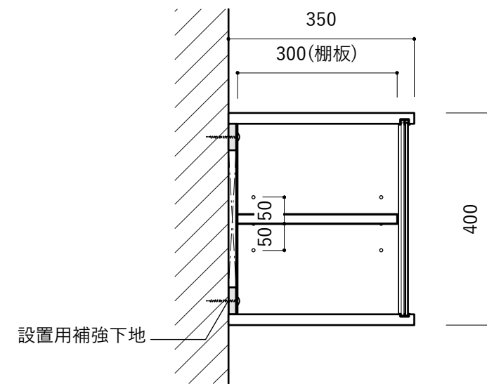
縦断面図
