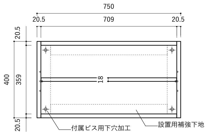
横断面図
