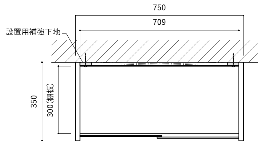
平断面図
